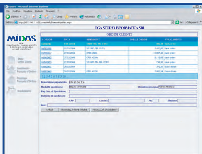
Interfaccia grafica
